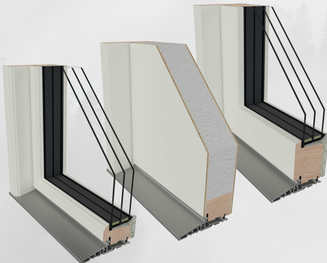
Eksempel på vinduesdør, pladedør og rammedøre.
